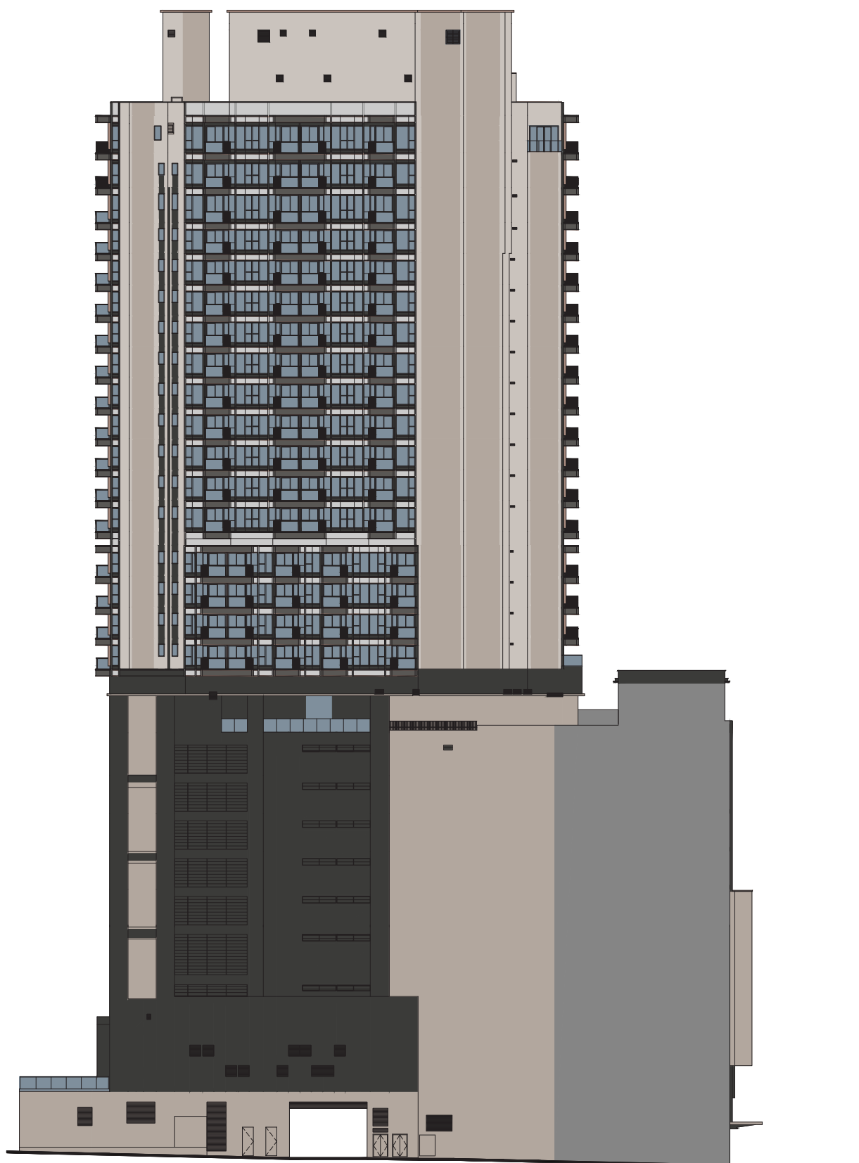
ELEVATION 3 立面 3
