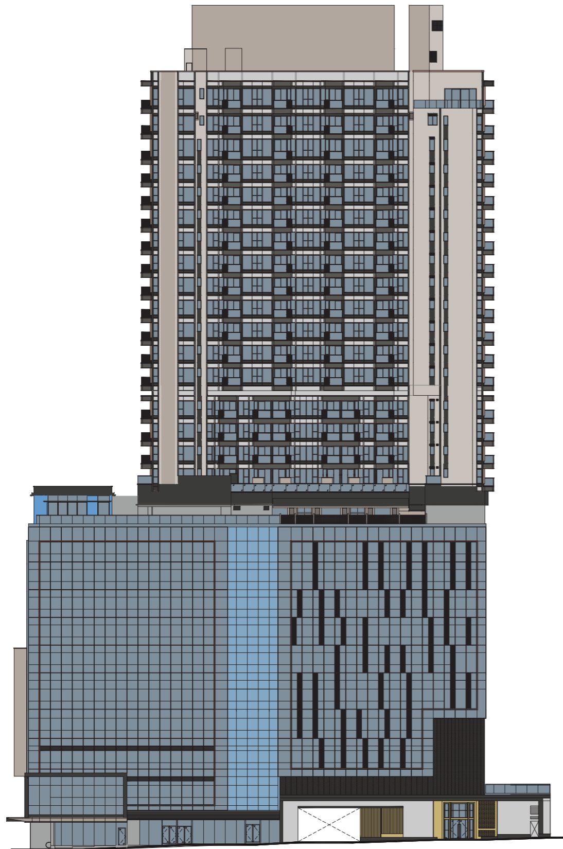
ELEVATION 1 立面 1
